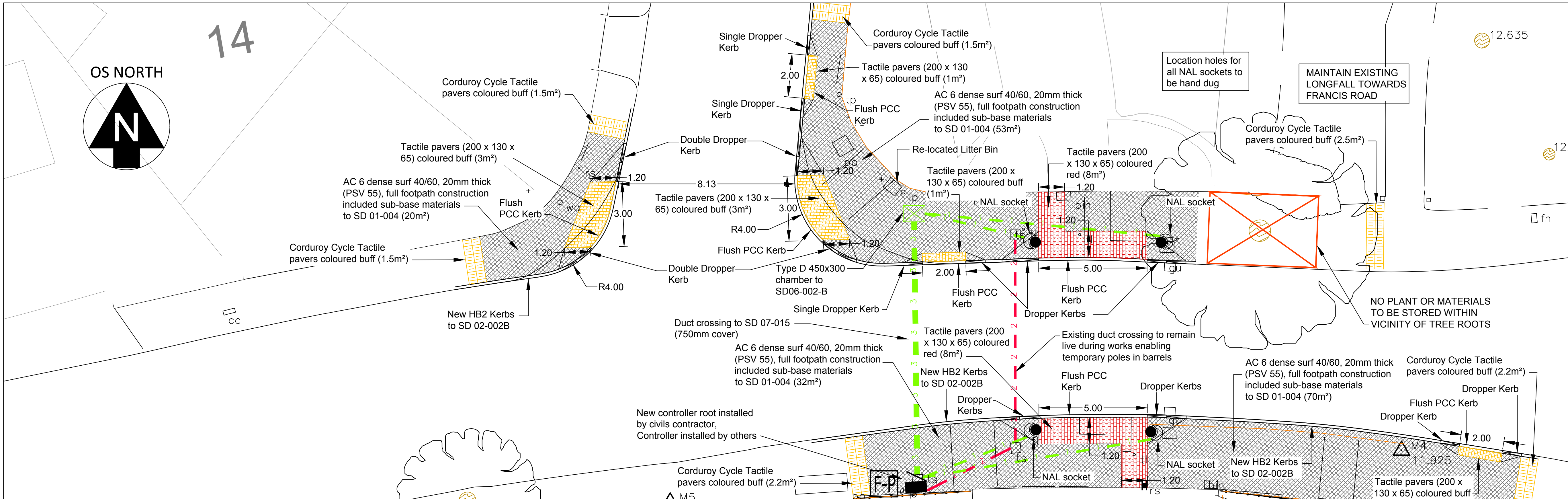
CONSTRUCTION PLAN 1:100 @A1
